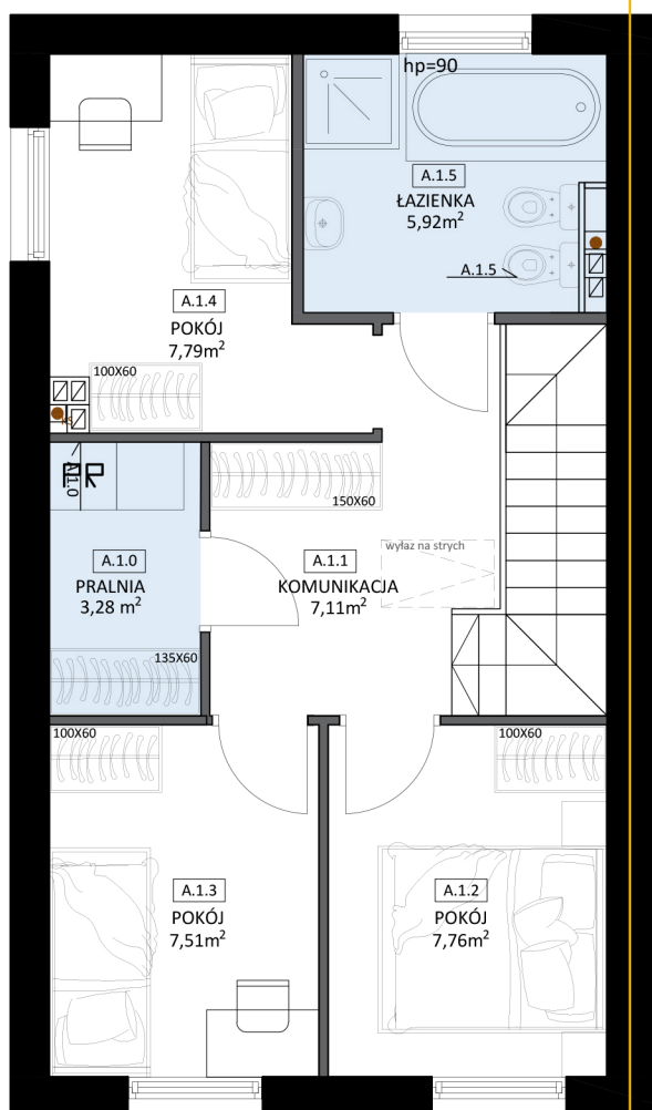
LOKAL A piętro
